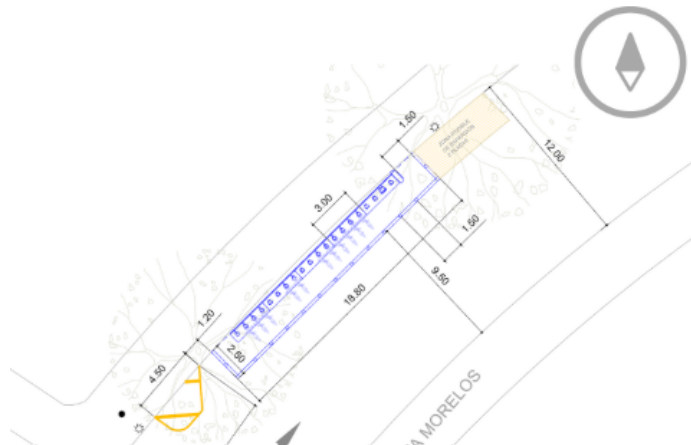
Plano 1. Especificaciones requeridas para la instalación de bolardos por estación.
